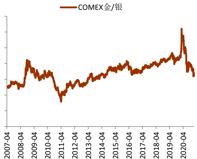
图表 10 COMEX 金银比价变化
